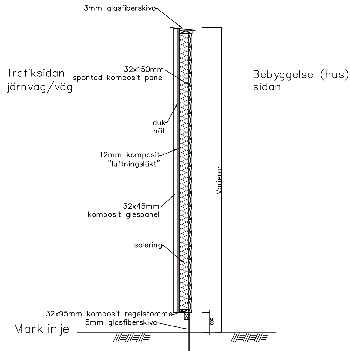
Sektion SKALA 1:25
