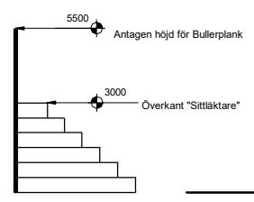
1 Sektion 1 : 100
