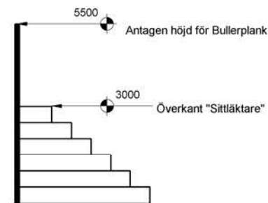
3 Sektion 1 : 100
